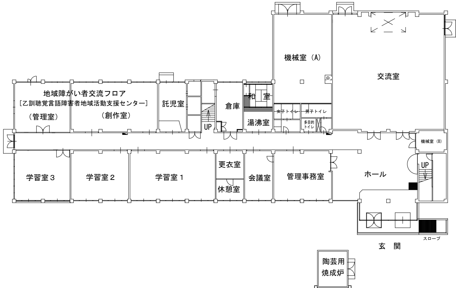
平面図 (1階)
