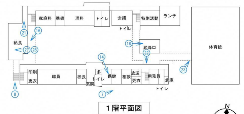
長岡第三小学校現況平面図 S=1/1000
