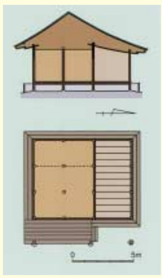
庵室の復元図
