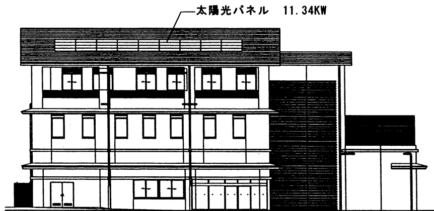
南立面図
