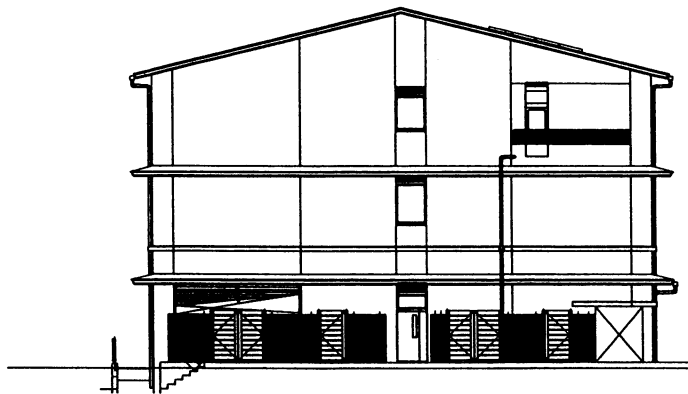
西立面図
