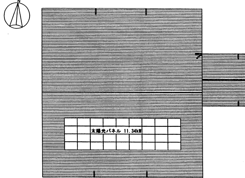
屋根伏図
