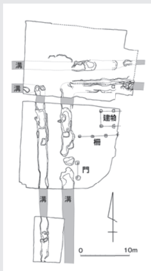
▲直交する溝と周辺施設
