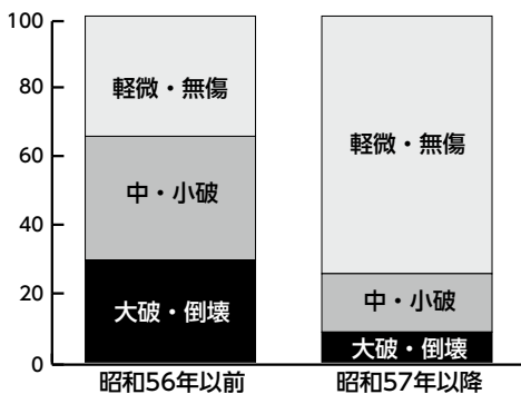
阪神大震災での被害状況(建築年別)
