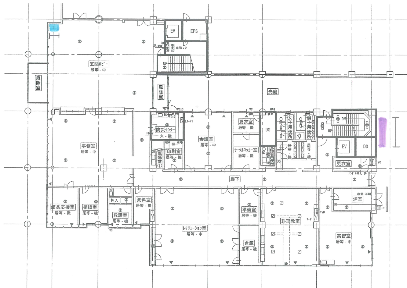
1階平面図 1/200
