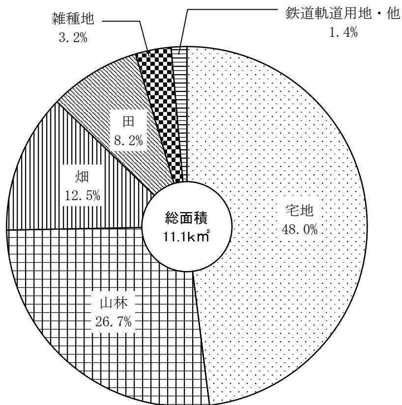
地目別土地面積（令和7年1月1日現在）
