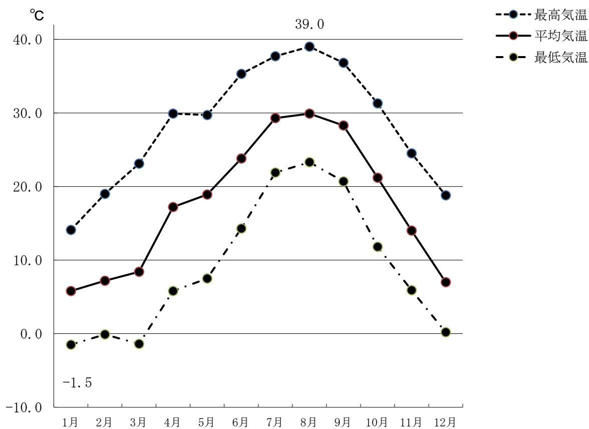
気 温 （令和6年中）
